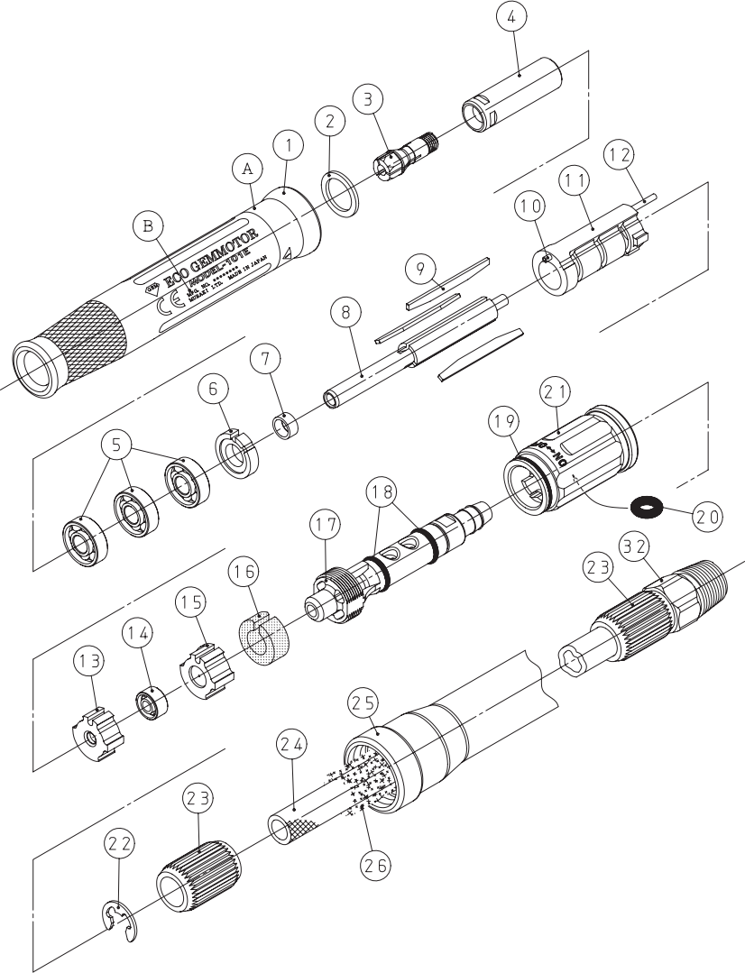
エコゼムモータMODEL-101E分解図
