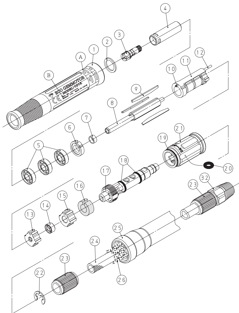
ゼムニューモータ モデル - 101分解図
