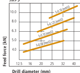
推力
