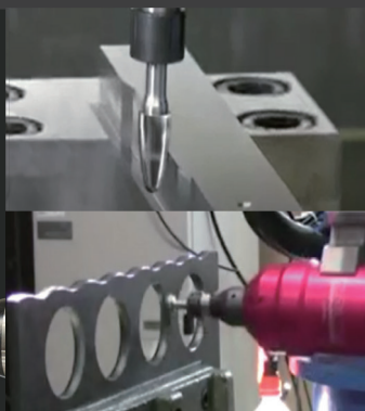
※画像提供 カトウ工機株式会社 DBR7-P型バリ取りホルダ
